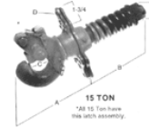
Spring Pintle Hook 15 & 25 Ton
